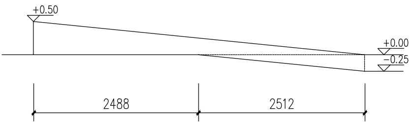
东侧地磅基础
