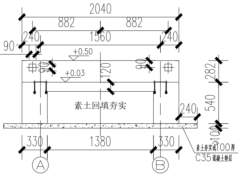
2—2 剖面图 1:50
