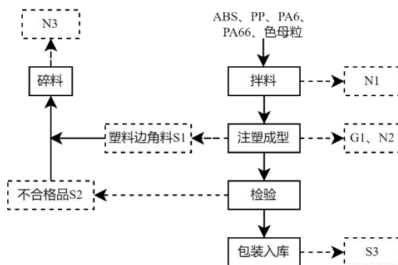
图4 电动工具塑料配件生产工艺流程及产污环节示意图
