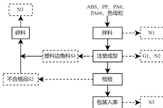
图3 项目生产工艺流程及产污节点图
