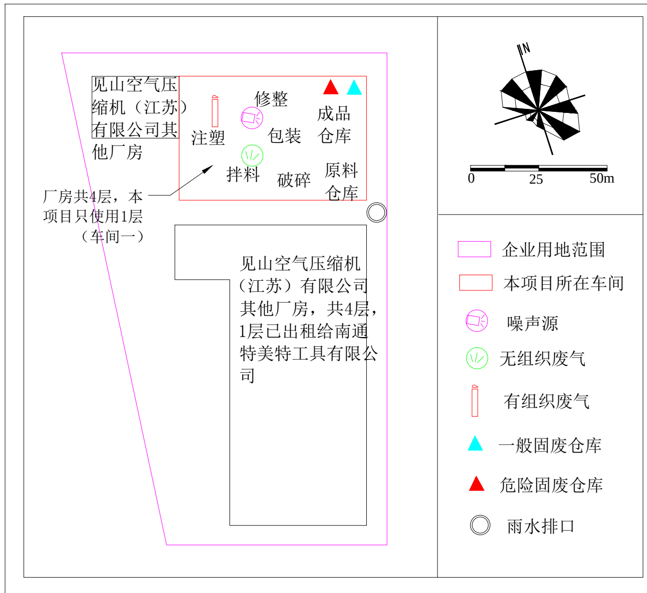
附图5 建设项目厂区平面布置图
