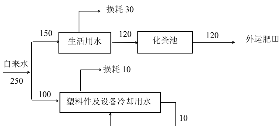
图 2-1 建设项目水平衡图 t/a
