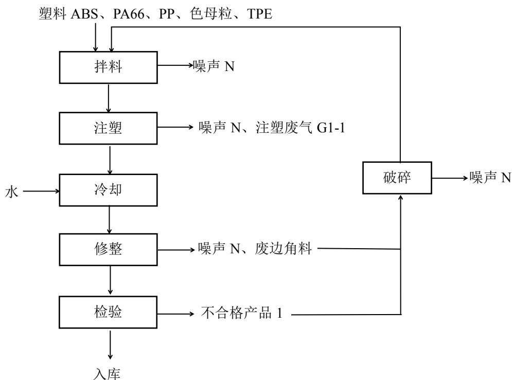
图 2-2 电动工具配件生产工艺流程及产污环节图
