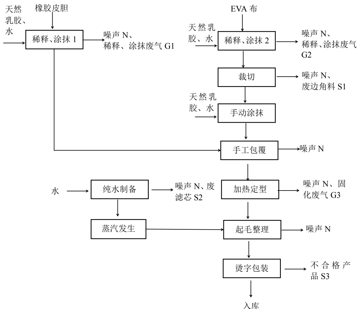
图 2-2 网球生产工艺流程图
