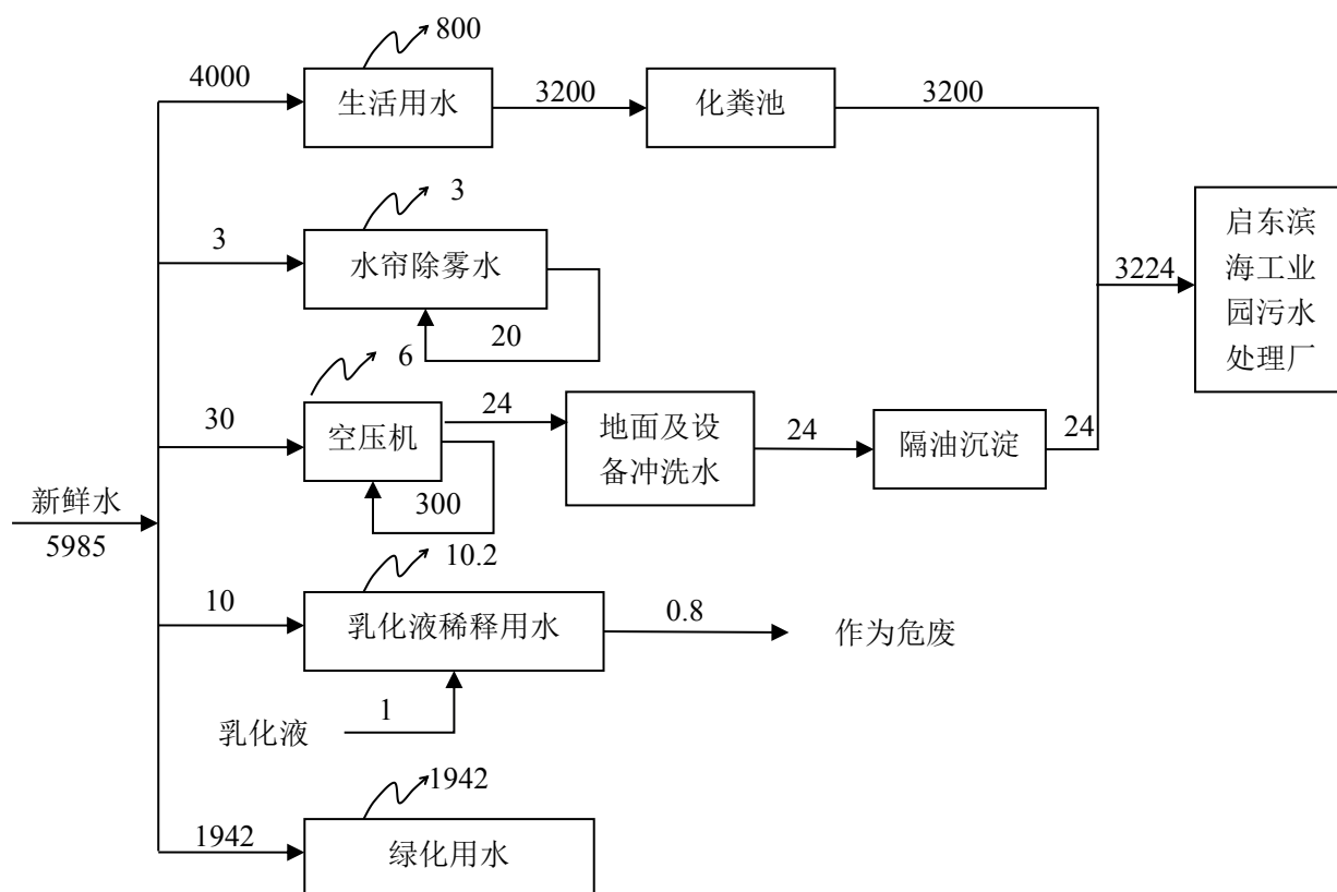
图 5-3 本项目建成后全厂水平衡图 (t/a)
