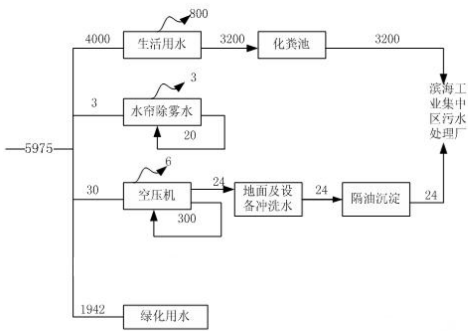
图 1-2 企业现有水平衡图 (t/a)
