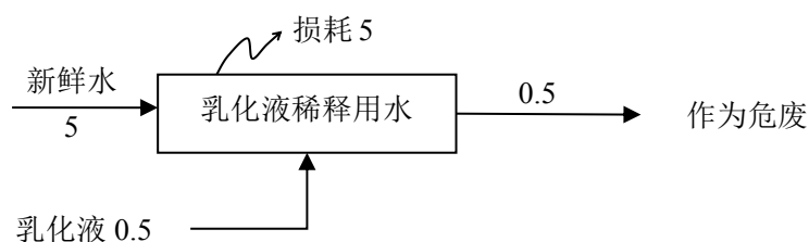
图 5-2 本项目水平衡图（t/a）
