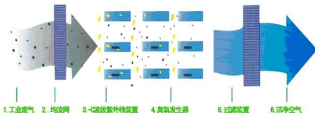
图 5-4 UV 光氧装置的工艺流程图
