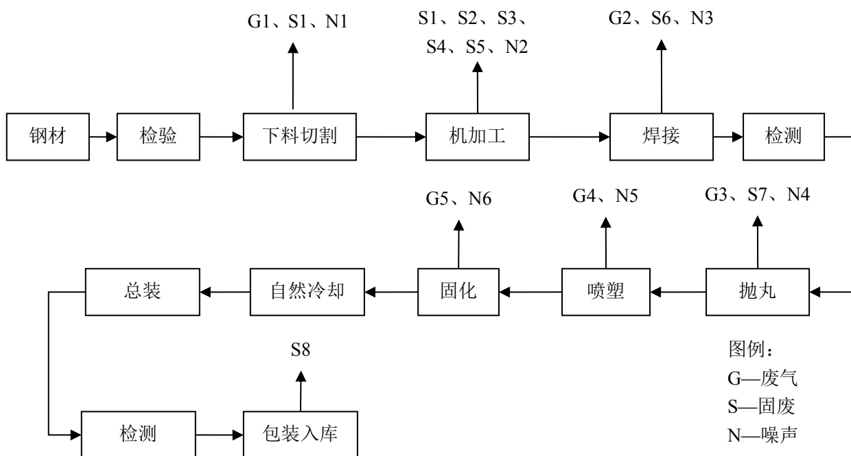
图 5-1 生产工艺流程及产排污节点图
