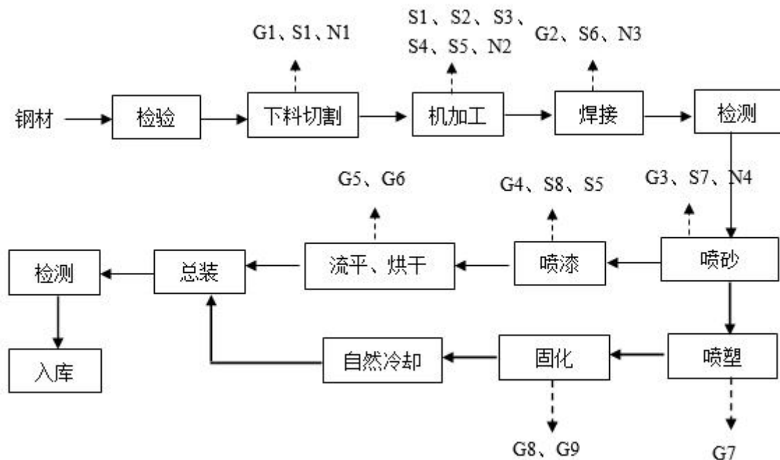
图 1-1 生产工艺流程图
