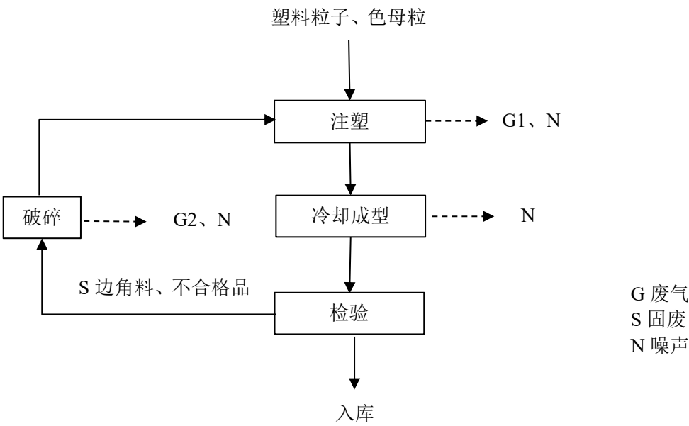
图 2-2 生产工艺流程及产污环节图
