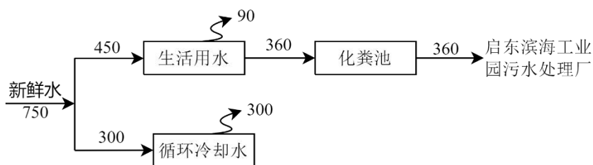
图 1 本项目水平衡图 (t/a)
