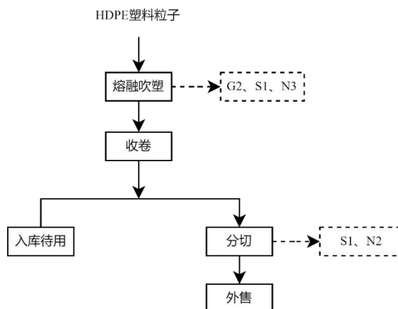
图 3 项目 HDPE 膜生产工艺流程及产污节点图
