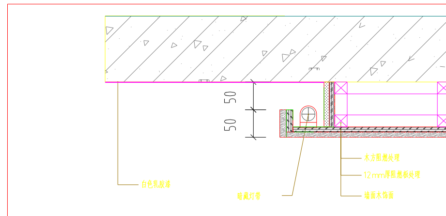
04 会议室墙面节点图 SCALE 1:50
