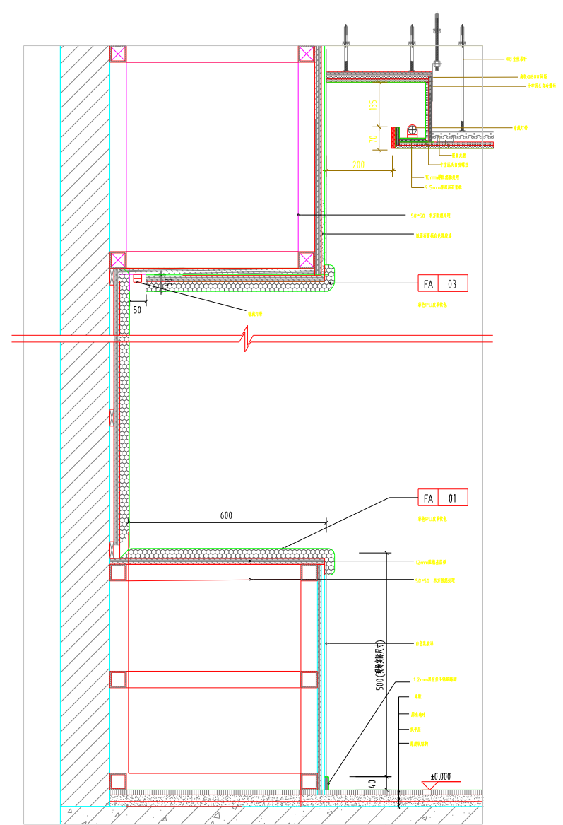
06 走道墙面节点图 SCALE 1:50
