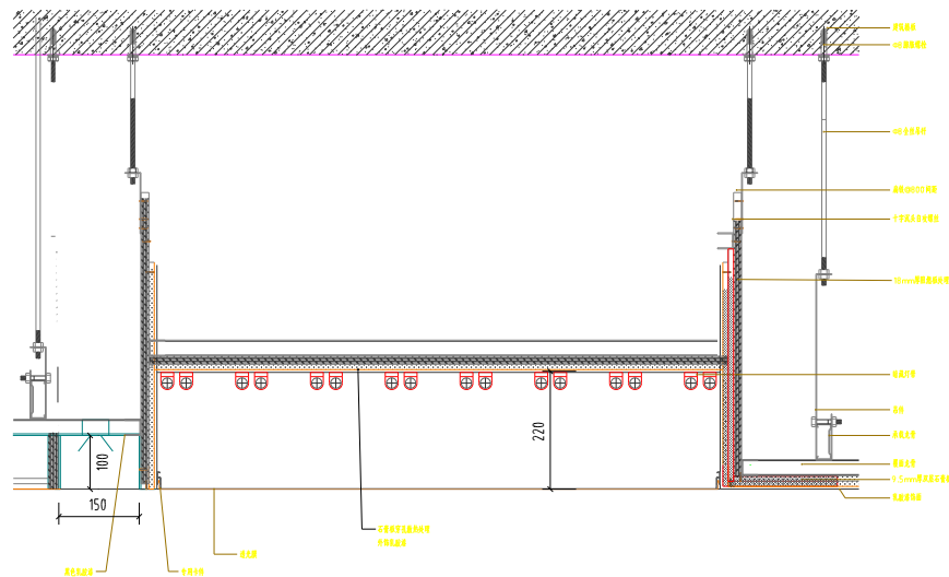
01 会议室天花软膜节点
