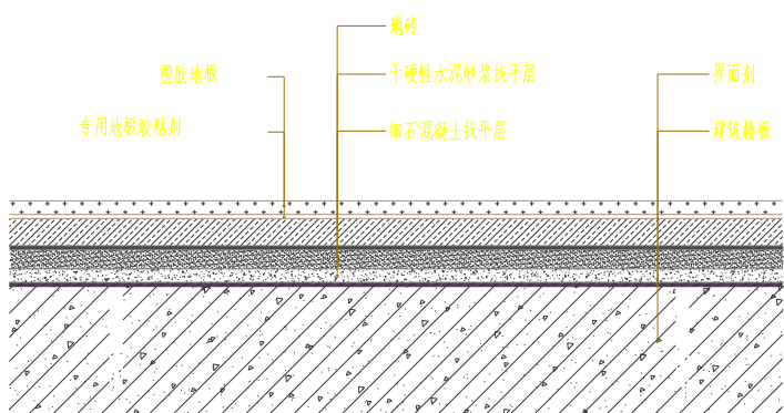
06 塑胶地板地坪节点图 SCALE 1:50
