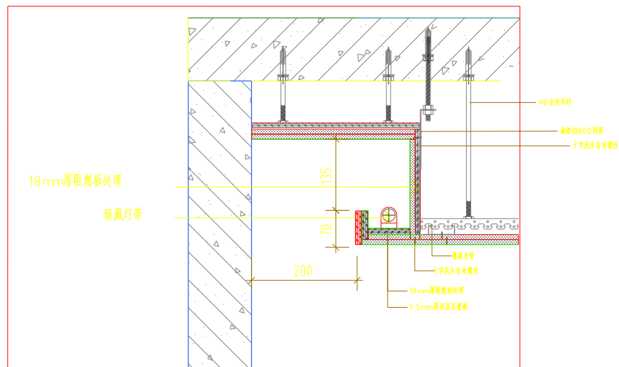
03 走道反光灯槽节点图 SCALE 1:50 走道
