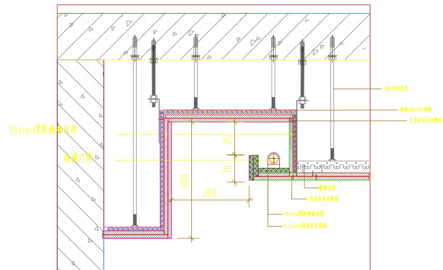
02 休闲室天花软膜节点 SCALE 1:50
