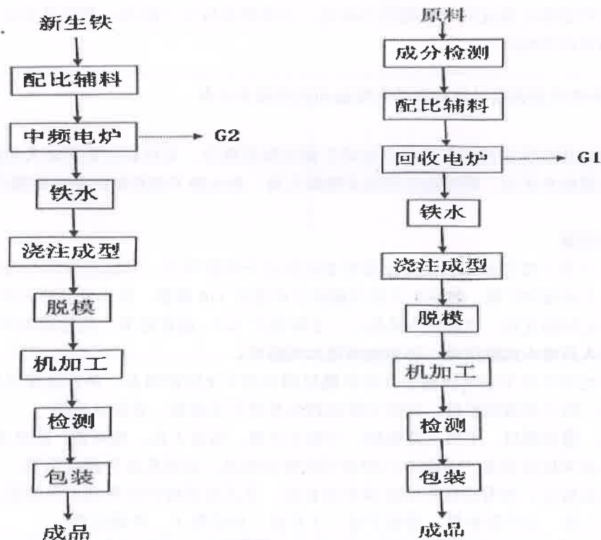
处理工艺流程图
