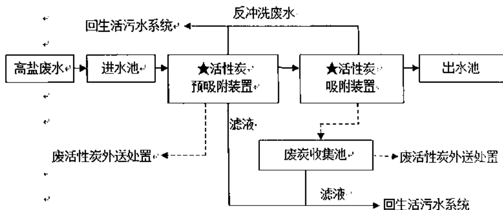
图 1 高盐废水处理工艺流程图
