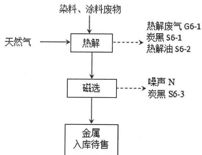
染料、涂料废物热解生产工艺图
