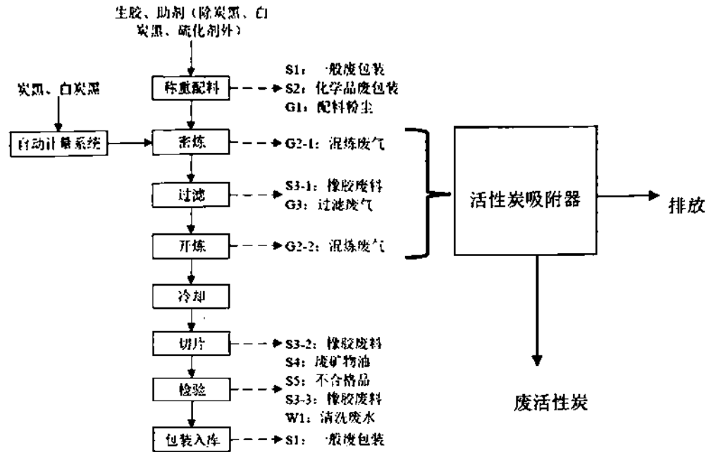
图 5.1-1 橡胶一次胶生产工艺流程
