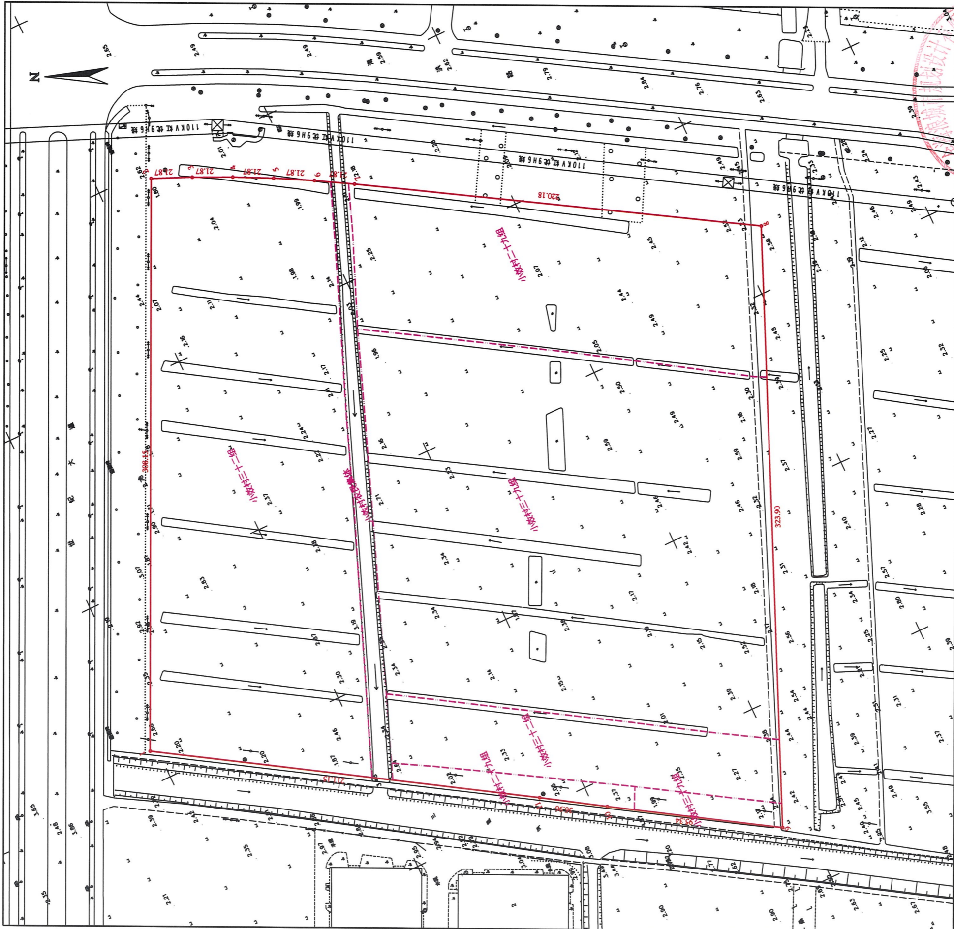
勘测定界图
