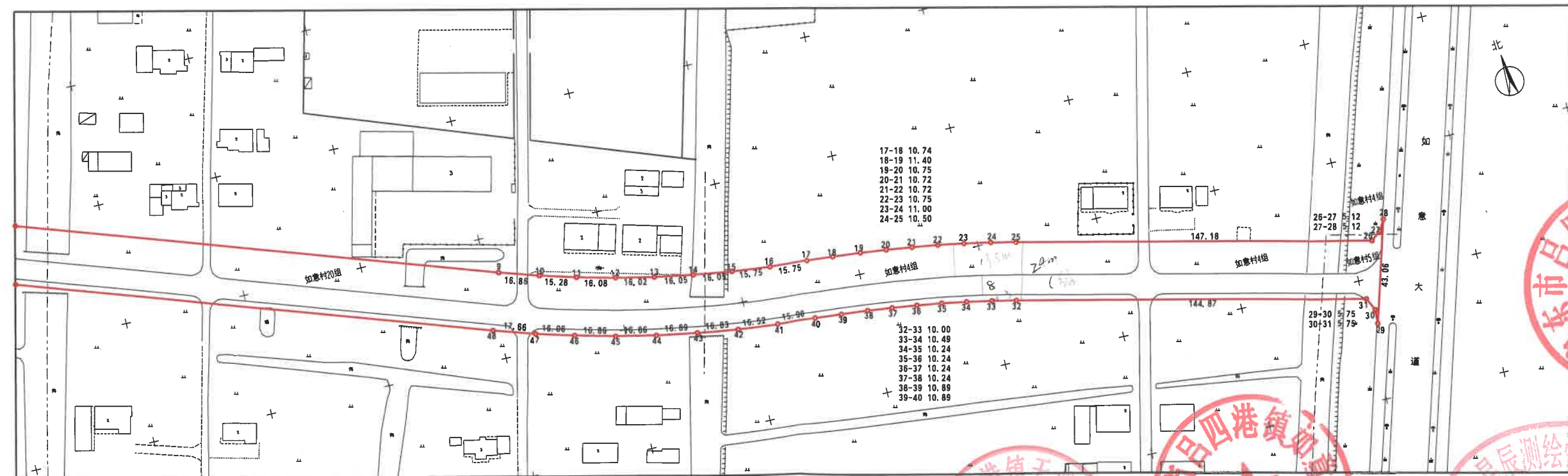
勘测定界图二
