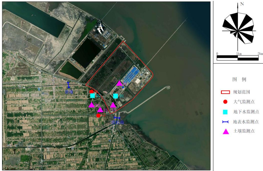
附图3 大气、土壤、地下水、地表水监测布点图
